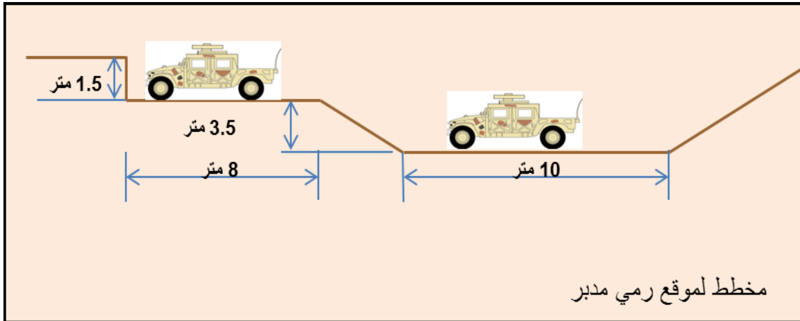
الشكل (13) موقع رمي مجهز
