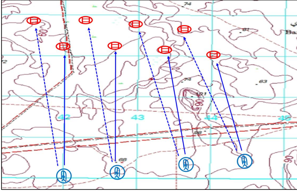
الشكل (23) نمط النار في العمق
