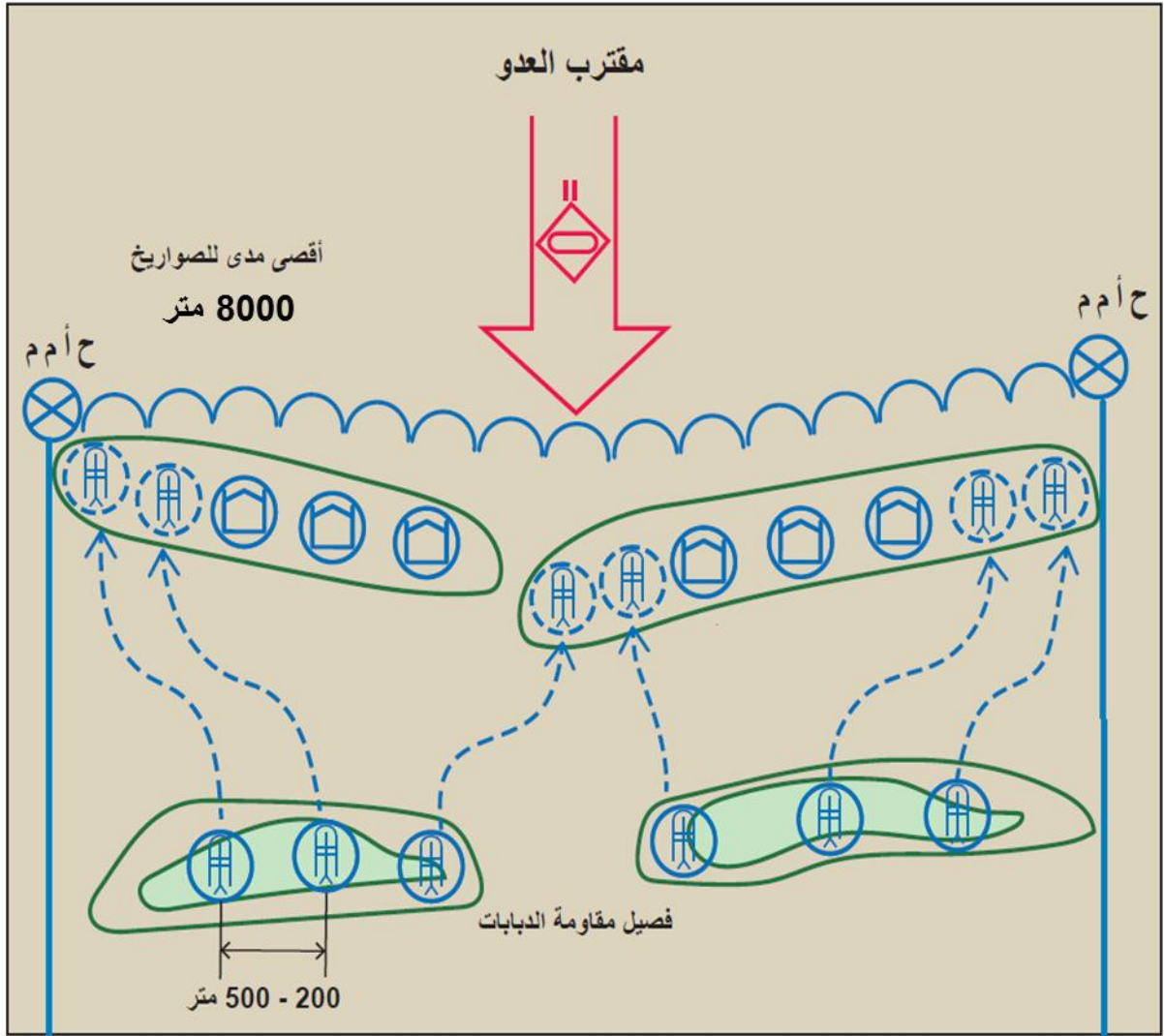
الشكل (14) مواقع قتال السرية والفصيل
