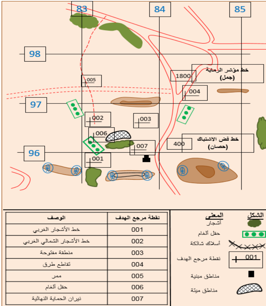
الشكل (28) خطة نيران فصيل مقاومة الدبابات على الخارطة
