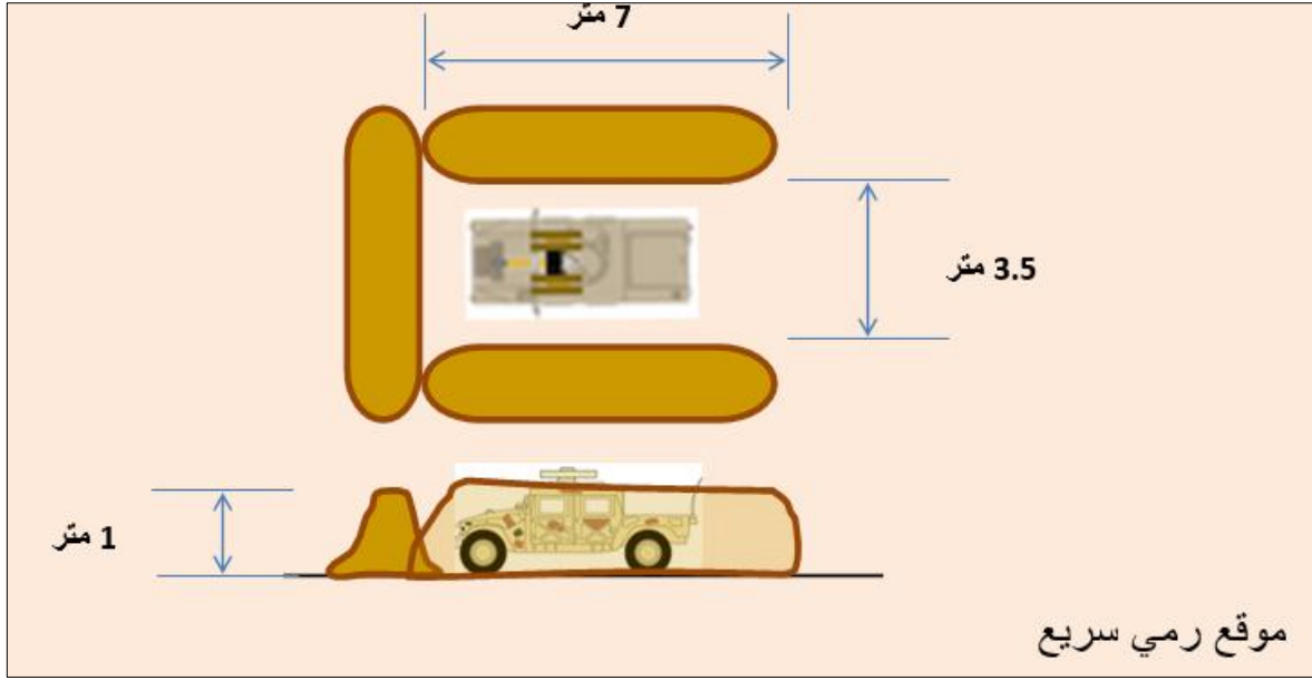
الشكل (12) موقع رمي سريع
