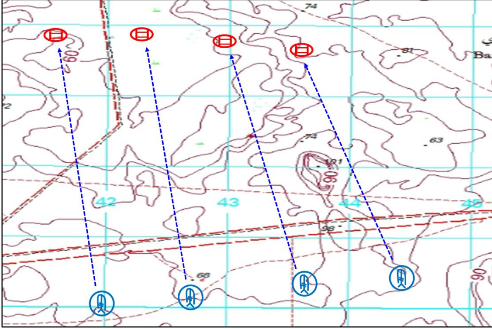
الشكل (21) نمط النار الجبهوية
