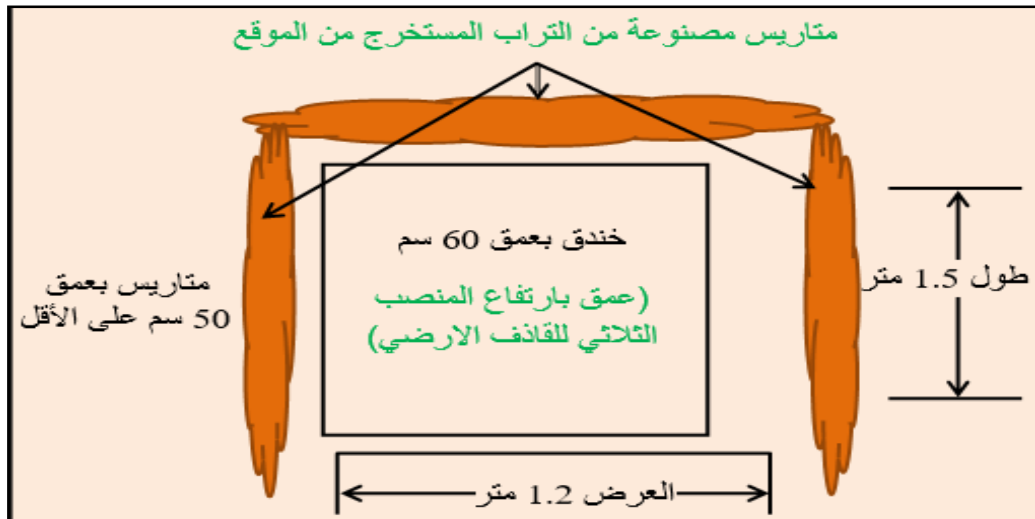
الشكل (29) موقع رمي لصاروخ مقاومة دبابات غير محمول
