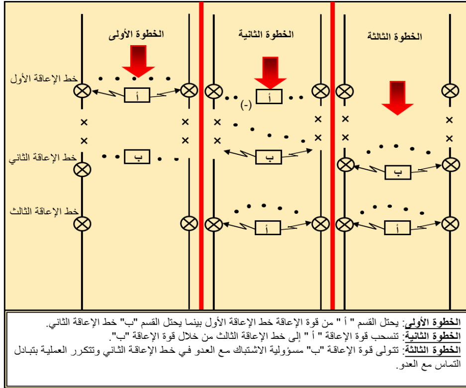
الشكل (32) الإعاقة من المواقع التبادلية
