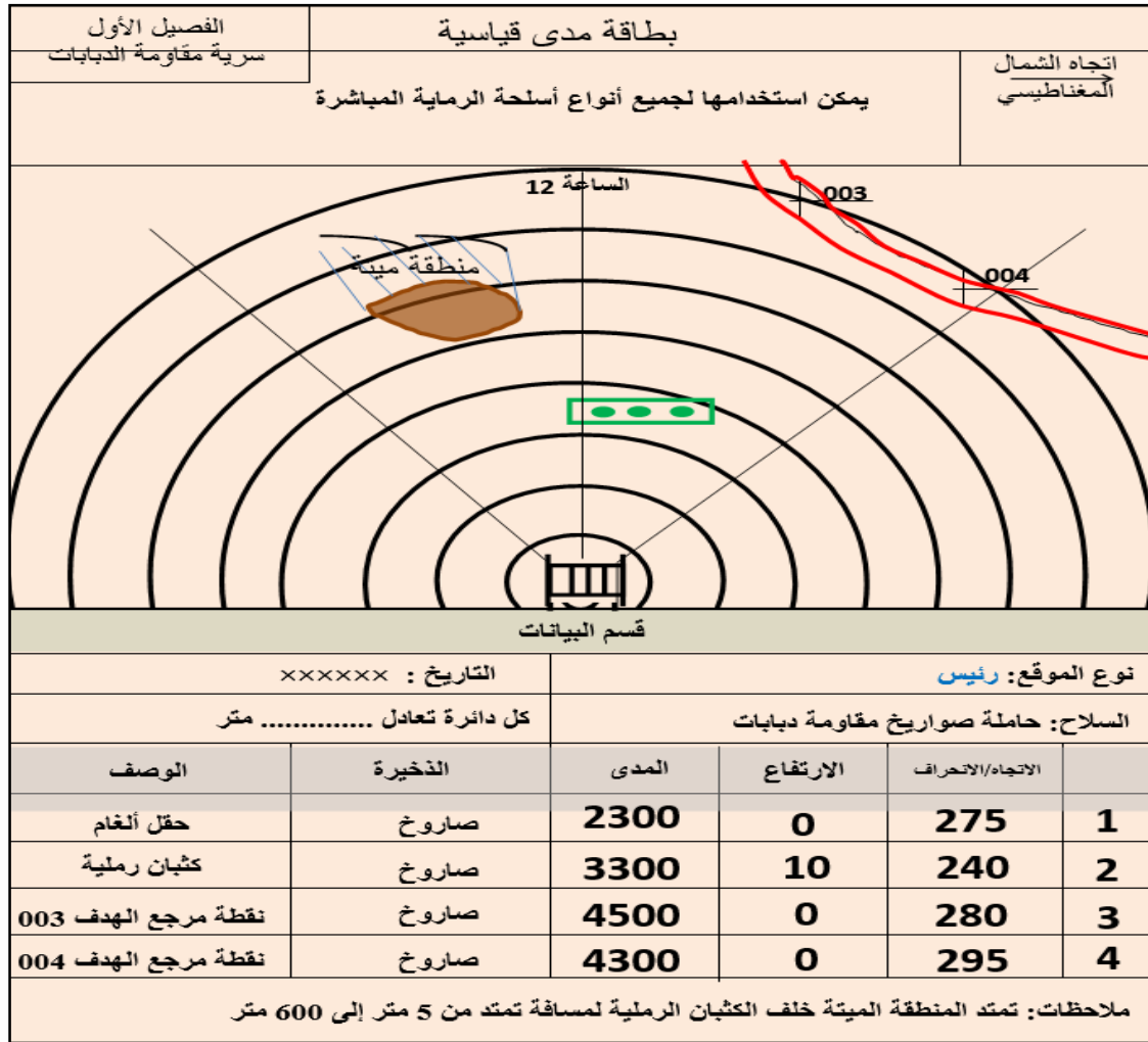
الشكل (27) بطاقة مدى قياسية
